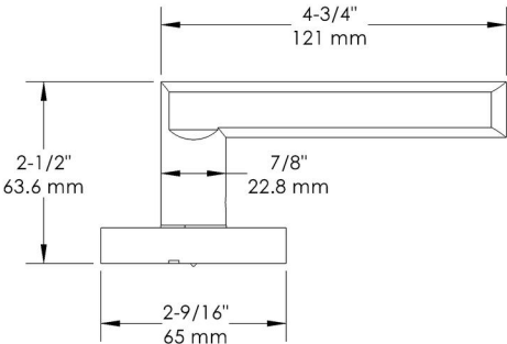
DIMENSIONS
